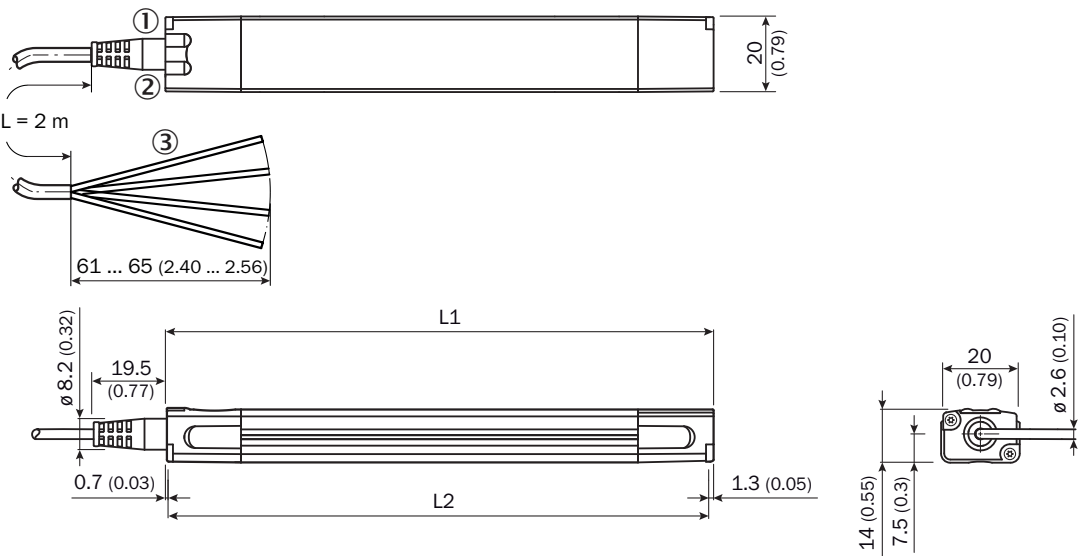
Rysunek wymiarowy Przewód
