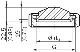
Rysunek wymiarowy Króciec z kołnierzem (DIN 11864-1) typu A z rowkową nakrętką kołpakową
