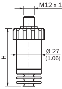
Rysunek wymiarowy Obudowa z wtykiem okrągłym M12 x 1, IP67
