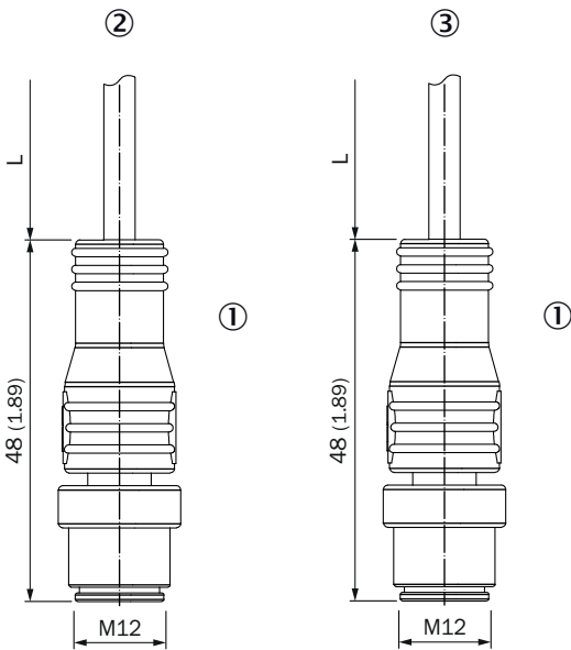
rysunek wymiarowy, przyłącze
