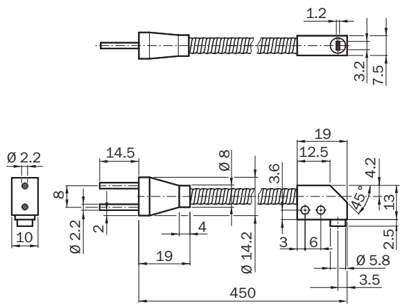
Rysunek wymiarowy LL3-LM37450
