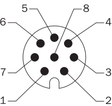
widok wtyczki urządzenia M12 na enkoderze
