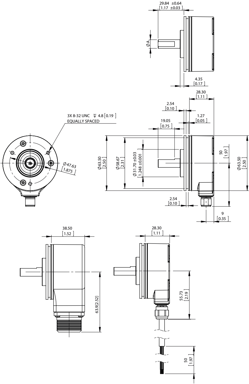
Rysunek wymiarowy Mocowanie na serwołożnierzu DFS25, wtyk promieniowy M12 i MS, wyprowadzenie przewodu
