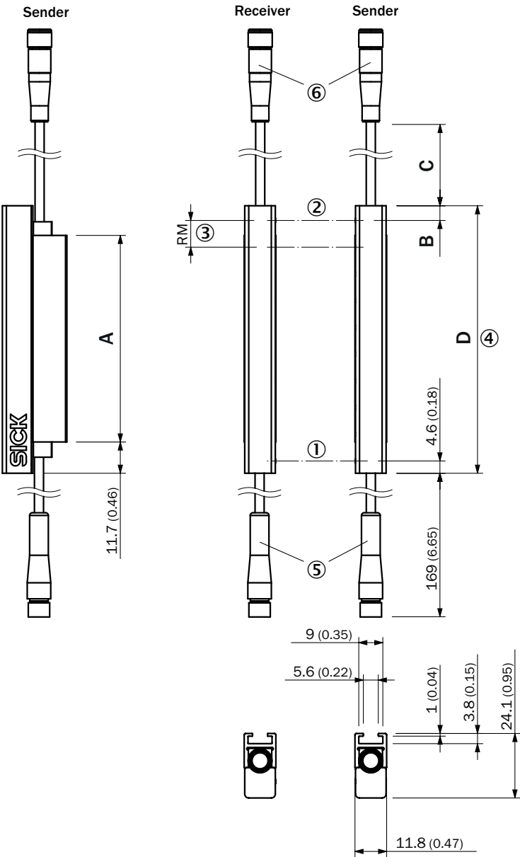
Rysunek wymiarowy SLGxxx-xxxFxxxxxx
