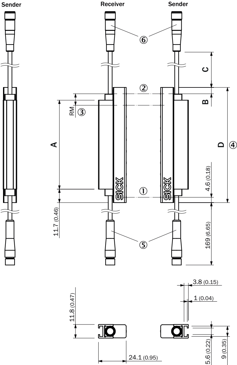
Rysunek wymiarowy SLGxxx-xxxSxxxxxxx
