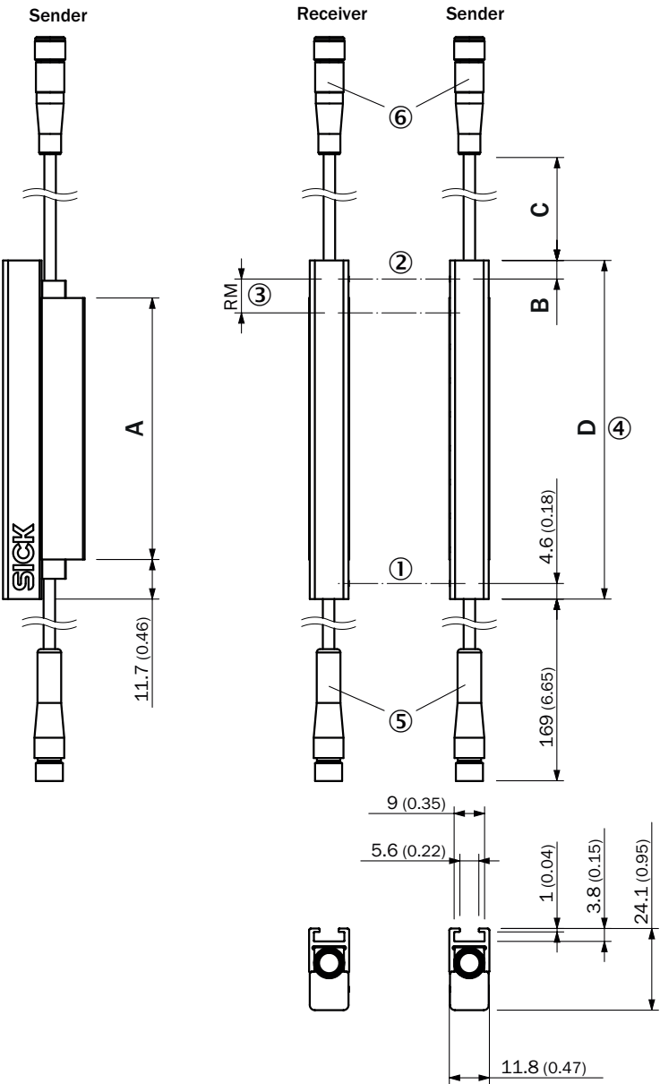
Rysunek wymiarowy SLGxxx-xxxFxxxxxx
