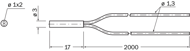
Rysunek wymiarowy
