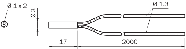
Rysunek wymiarowy LL3-DK04
