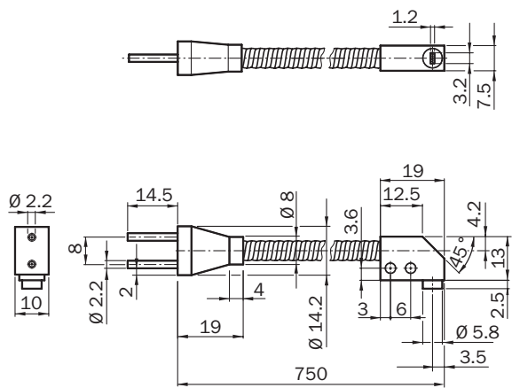
Rysunek wymiarowy LL3-LM37750
