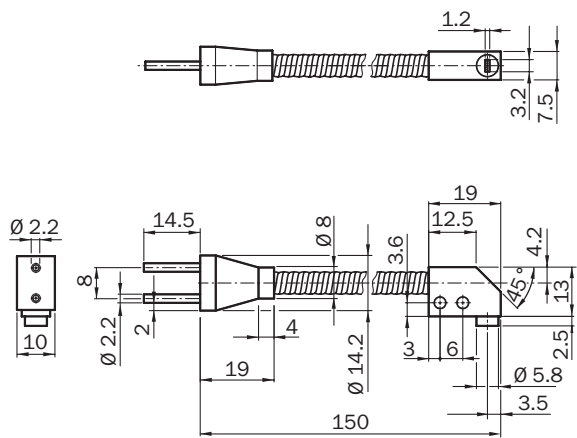
Rysunek wymiarowy LL3-LM37150
