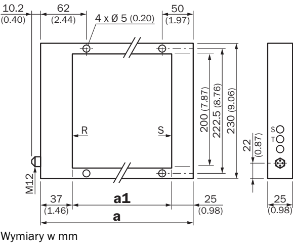
Rysunek wymiarowy FLGx-200xxx1x
