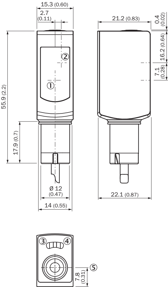
Rysunek wymiarowy WTB4SL-3, przewód
