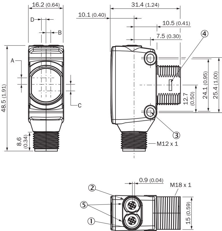
Rysunek wymiarowy
