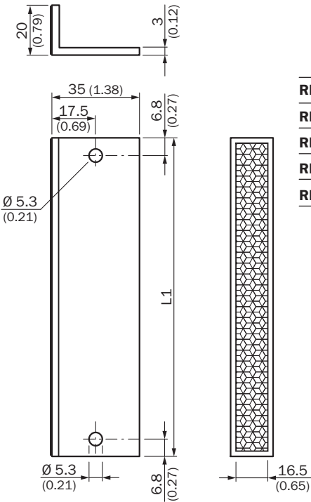
Wymiary w mm
