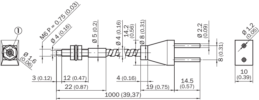
Rysunek wymiarowy LL3-DW01
