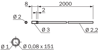
Rysunek wymiarowy LL3-TR10
