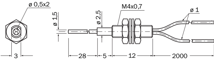
Rysunek wymiarowy
