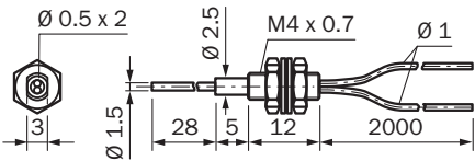
Rysunek wymiarowy LL3-DT05
