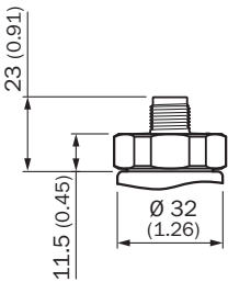
Wymiary w mm
