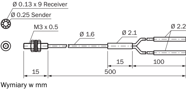
Rysunek wymiarowy LL3-DK21
