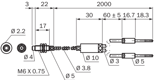
Rysunek wymiarowy LL3-DH03
