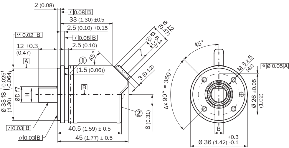
Rysunek wymiarowy Wałek, mocowanie na serwołożnierzu, przewód
