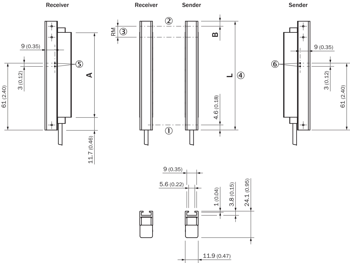
Rysunek wymiarowy, czujnik
