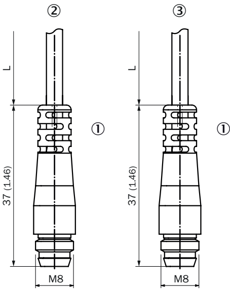
rysunek wymiarowy, przyłącze
