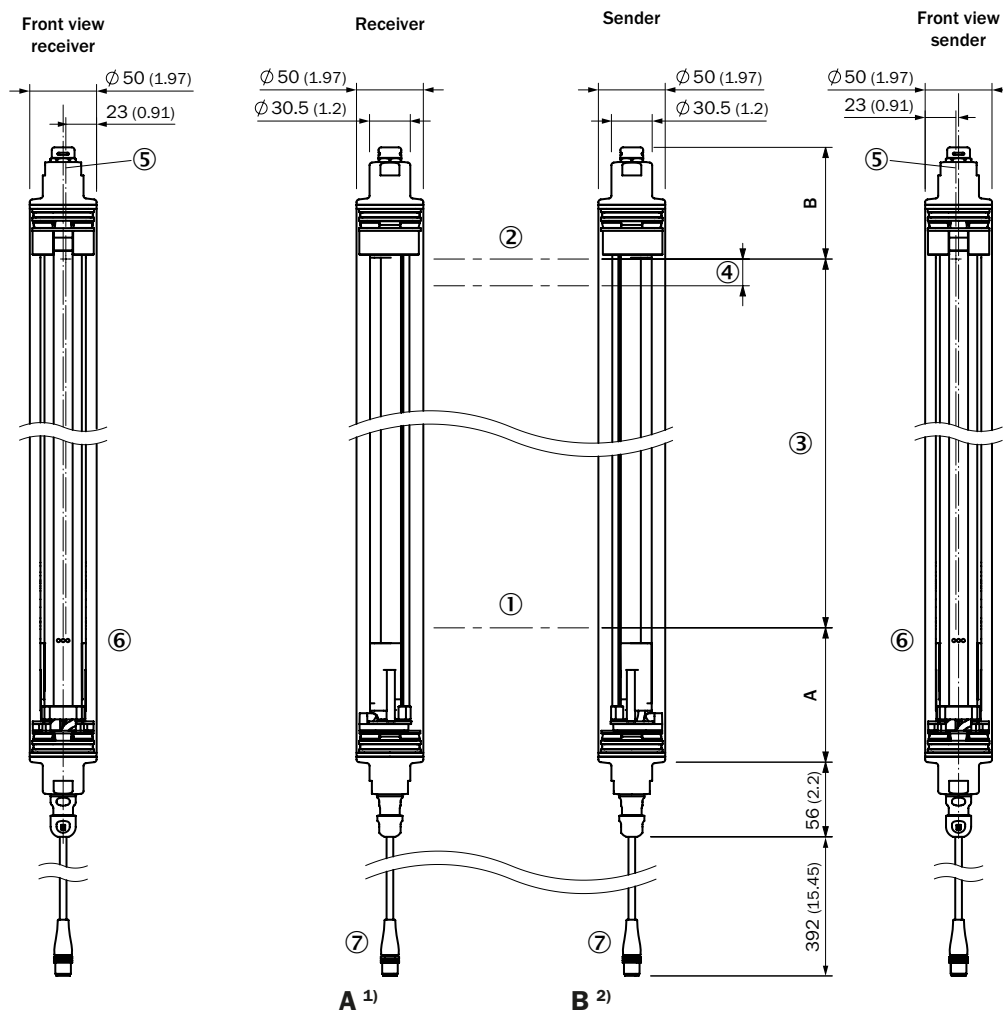
Rysunek wymiarowy
