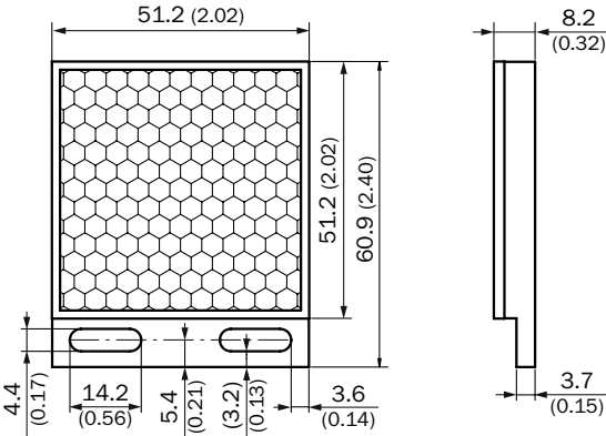
Rysunek wymiarowy
