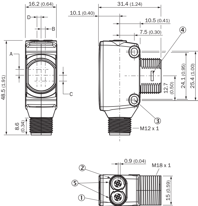
Rysunek wymiarowy
