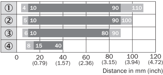
Wykres zasięgu wykrywania WTB2S-2, 110 mm
