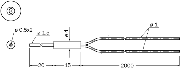
Rysunek wymiarowy
