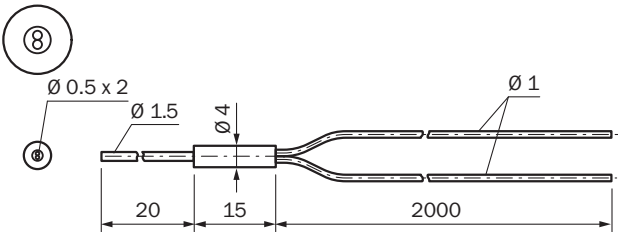
Rysunek wymiarowy LL3-DK43
