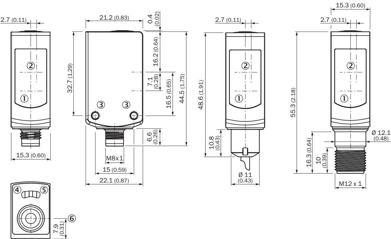
Rysunek wymiarowy WTB4SL-3, wtyk
