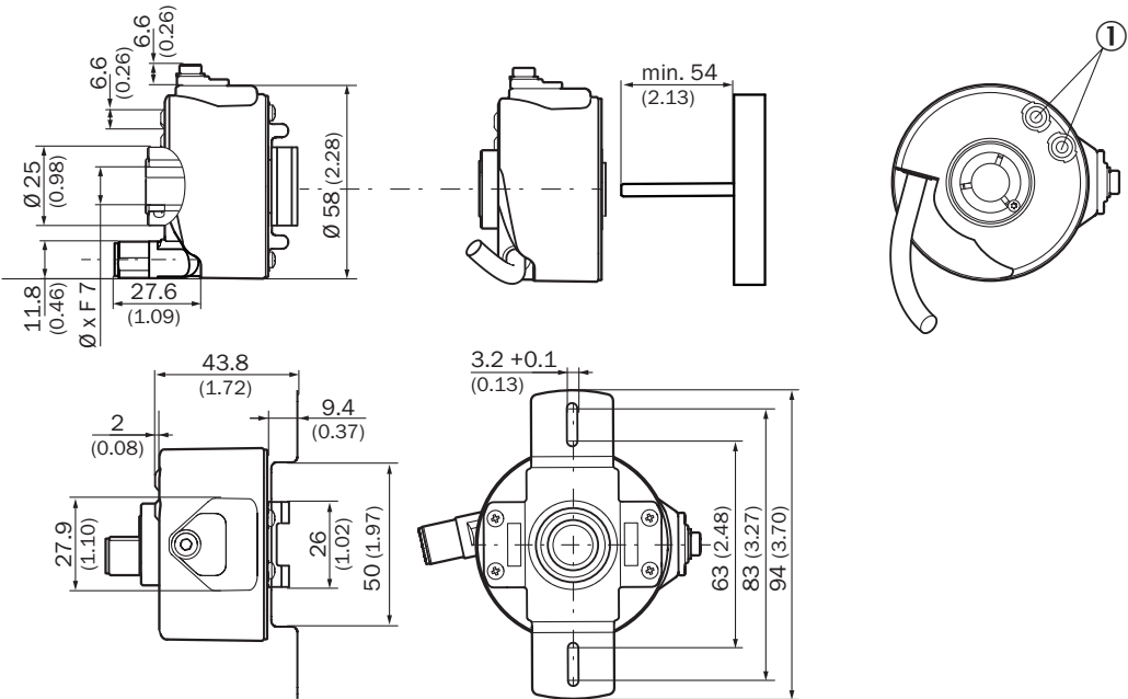
Rysunek wymiarowy Drażony wałek przetykany zaciskany z tyłu
