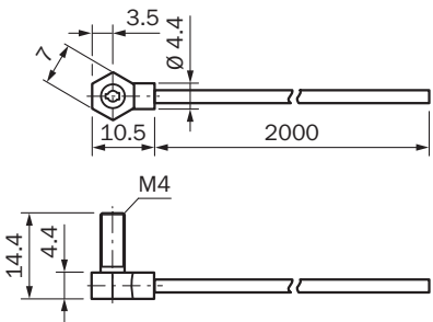
Rysunek wymiarowy LL3-TV05, LL3-TV06, LL3-TV07
