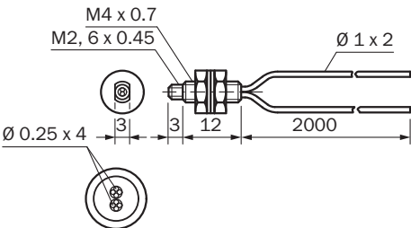
Rysunek wymiarowy LL3-DR06
