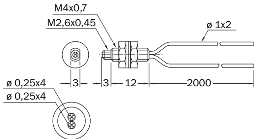
Rysunek wymiarowy
