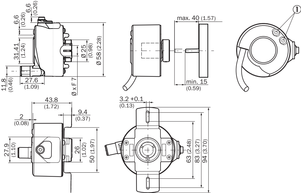
Rysunek wymiarowy Otwór nieprzelotowy
