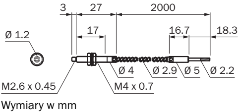
Rysunek wymiarowy LL3-TH08
