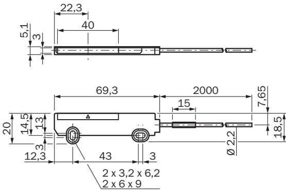
Rysunek wymiarowy LL3-TS40
