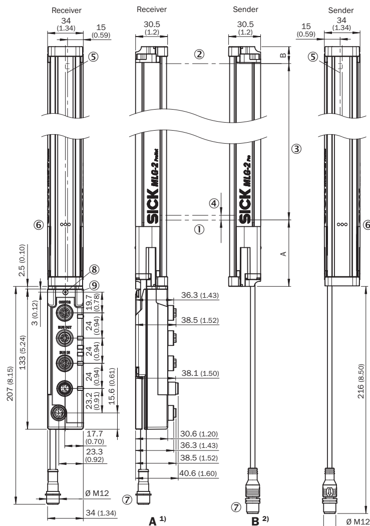
Rysunek wymiarowy
