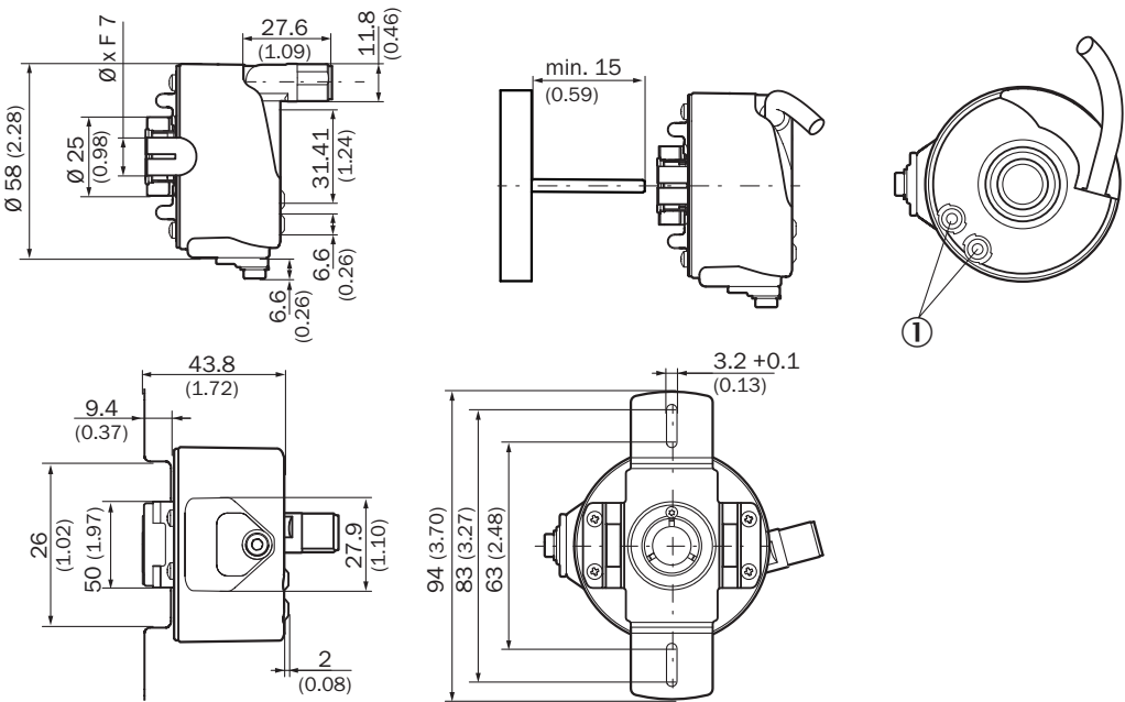
Rysunek wymiarowy Wersja z otworem przelotowym – zacisk z przodu
