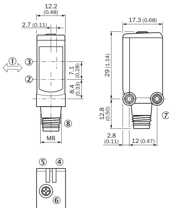
Rysunek wymiarowy WTB4SL-3, wtyk
