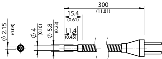
Rysunek wymiarowy LL3-LM31300
