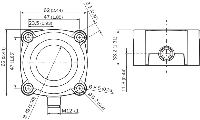
Rysunek wymiarowy | from serial number S/N 2405xxxx
