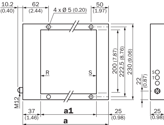
Rysunek wymiarowy FLGx-200xxx1x
