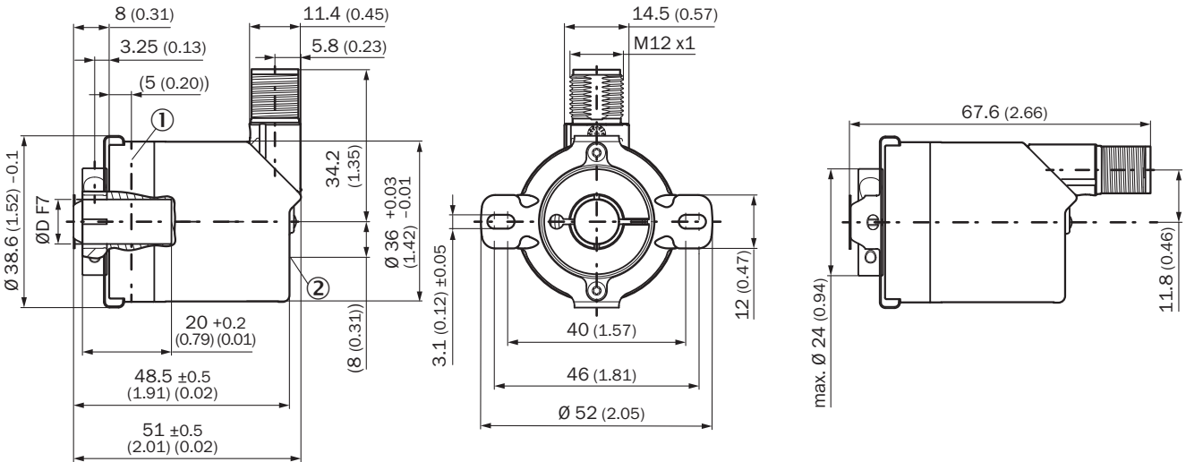
Rysunek wymiarowy Otwór nieprzelotowy, wtyk
