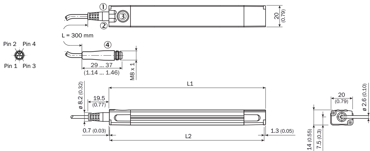
Rysunek wymiarowy Przewód z 4-biegunowym wtykiem M8
