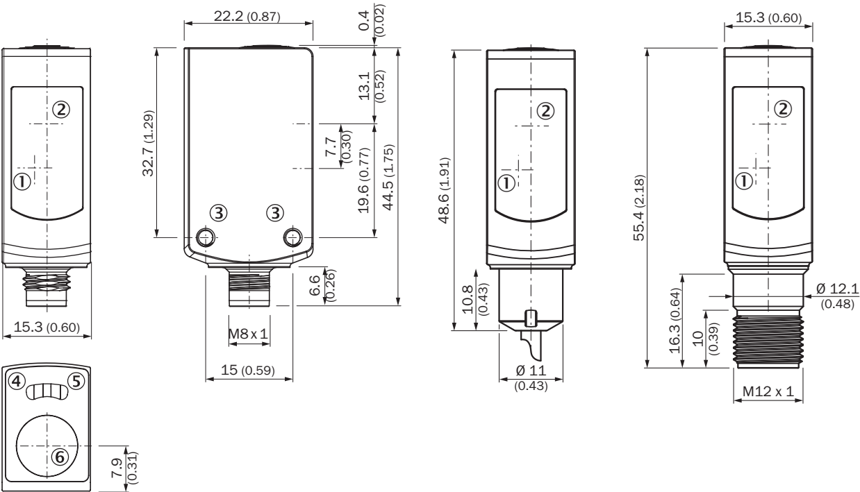
Rysunek wymiarowy WTB4S-3V, WTF4S-3V, z przyciskiem Teach-in
