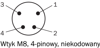
Wtyk M8, 4-pinowy, niekodowany
