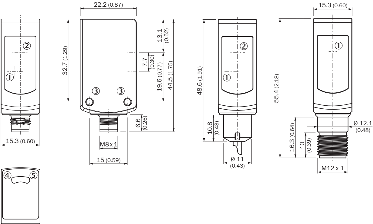
Rysunek wymiarowy WTB4S-3V, WTF4S-3V, bez przycisku Teach-in
