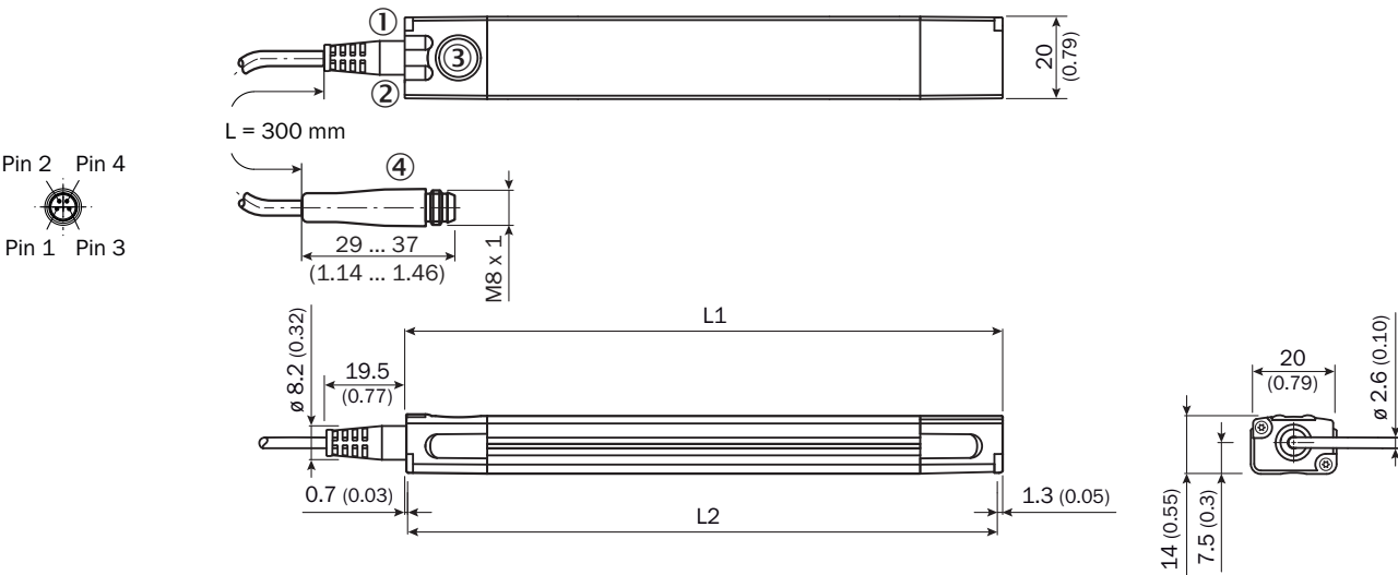
Rysunek wymiarowy Przewód z 4-biegunowym wtykiem M8
